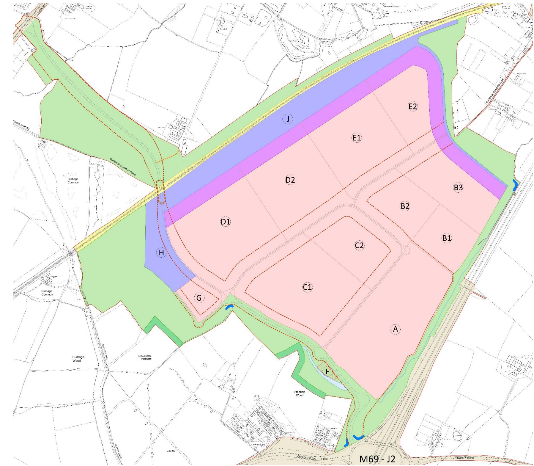
Fig 20. Parameters Plan – Area 2 of 5 and Zonal Parameters Table
